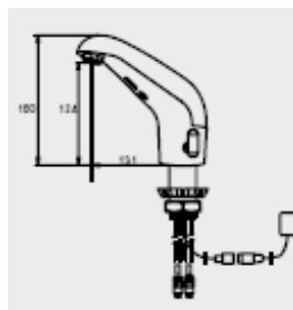
MA nr 72 00 73 Zasilanie poprzez zasilacz Napięcie 7,5 V. Wskaźnik braku napięcia.
