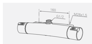
Duschblandare T5 Utlopp upp MA-nr 73 10 50 RSK-nr 834 40 66 MA-nr 73 10 50.0011 RSK-nr 834 40 67*
