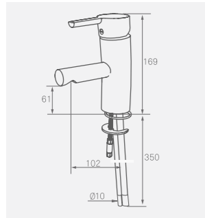
Tvättställsblandare B5 MA-nr 73 30 00.CA RSK-nr 834 45 02
