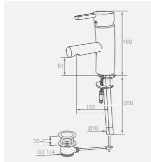
Tvättställsblandare B5 med lyftventil MA-nr 73 30 50.CA RSK-nr 834 45 06
