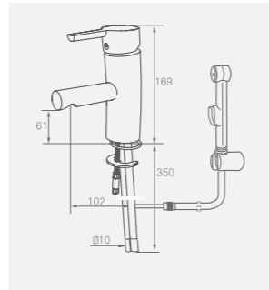
Tvättställsblandare B5 med självstängande handdusch MA-nr 73 30 05 RSK-nr 834 44 95 med lyftventil MA-nr 73 30 55 RSK-nr 834 45 11
