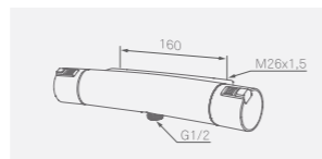
Duschblandare T5 Utlopp ned MA-nr 73 10 00 RSK-nr 834 40 62 MA-nr 73 10 00.0011 RSK-nr 834 40 63*
