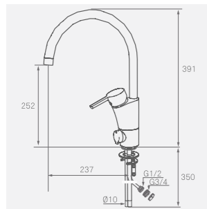
Köksblandare K5 Med diskmaskinsavstängning MA-nr 73 21 50 RSK-nr 831 83 91 Utan diskmaskinsavstängning MA-nr 73 21 00 RSK-nr 831 83 75
